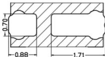
1-3 Bottom view 背视图
